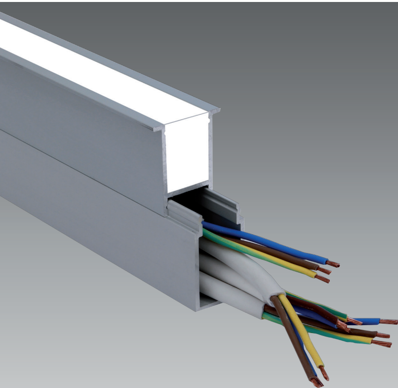
Beispiel für EA-3 mit Kabelkanal AKF-3 example for EA-3 with cable conduit AKF-3
